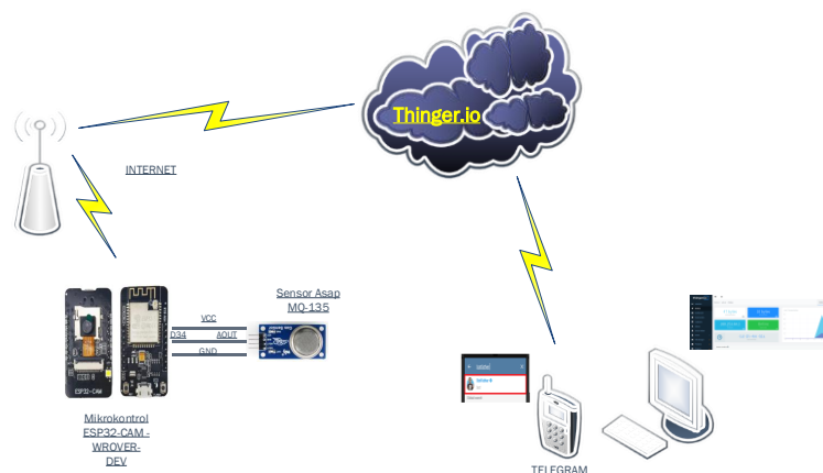
Gambar 4. Blok diagram system informasi deteksi dini polusi udara berbasis IoT
