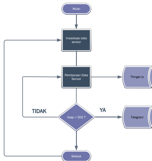
Gambar 10. Flow Chart program Peringatan Dini Polusi Udara dengan Sensor MQ-135 dan Pengiriman Notifikasi via Telegram Berbasis IoT
