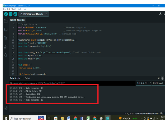
Gambar 8. Saat ambang batas \geq 200 ppm sitem kirim gambar foto dari ESP32 Cam
