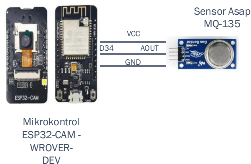
Gambar 3. Gambar rangkaian mikrokontrol ESP32Cam dengan sensor MQ135
