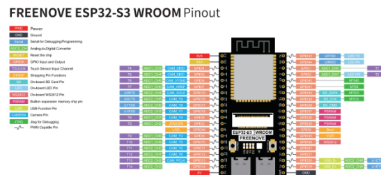
Gambar 1. Mikrokontrol ESP32-CAM
